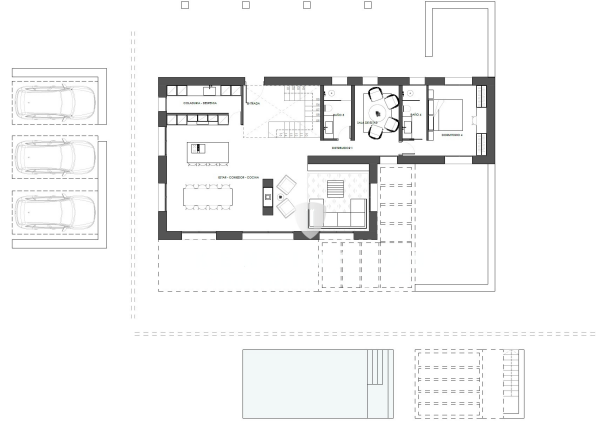
PLANTA BAJA (CERRA NUEVA)
