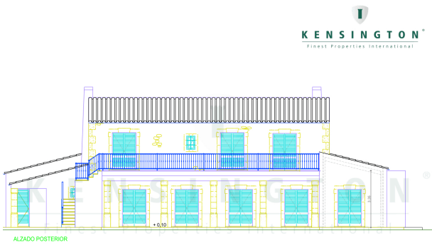
ALZADO POSTERIOR
